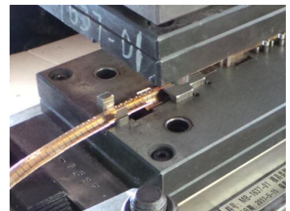
模具冲压一角
