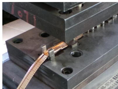
模具冲压一角
