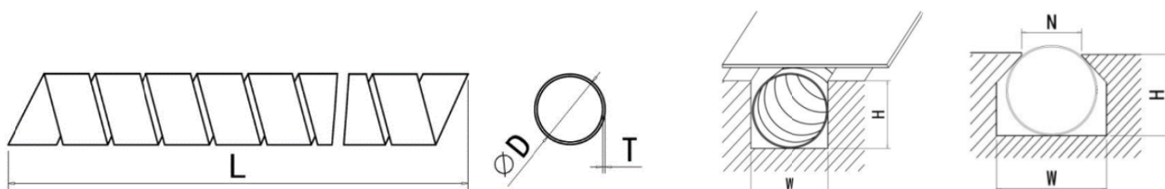
螺旋管尺寸参考图 I. 安装于标准O型槽中 II. 安装于燕尾槽中
